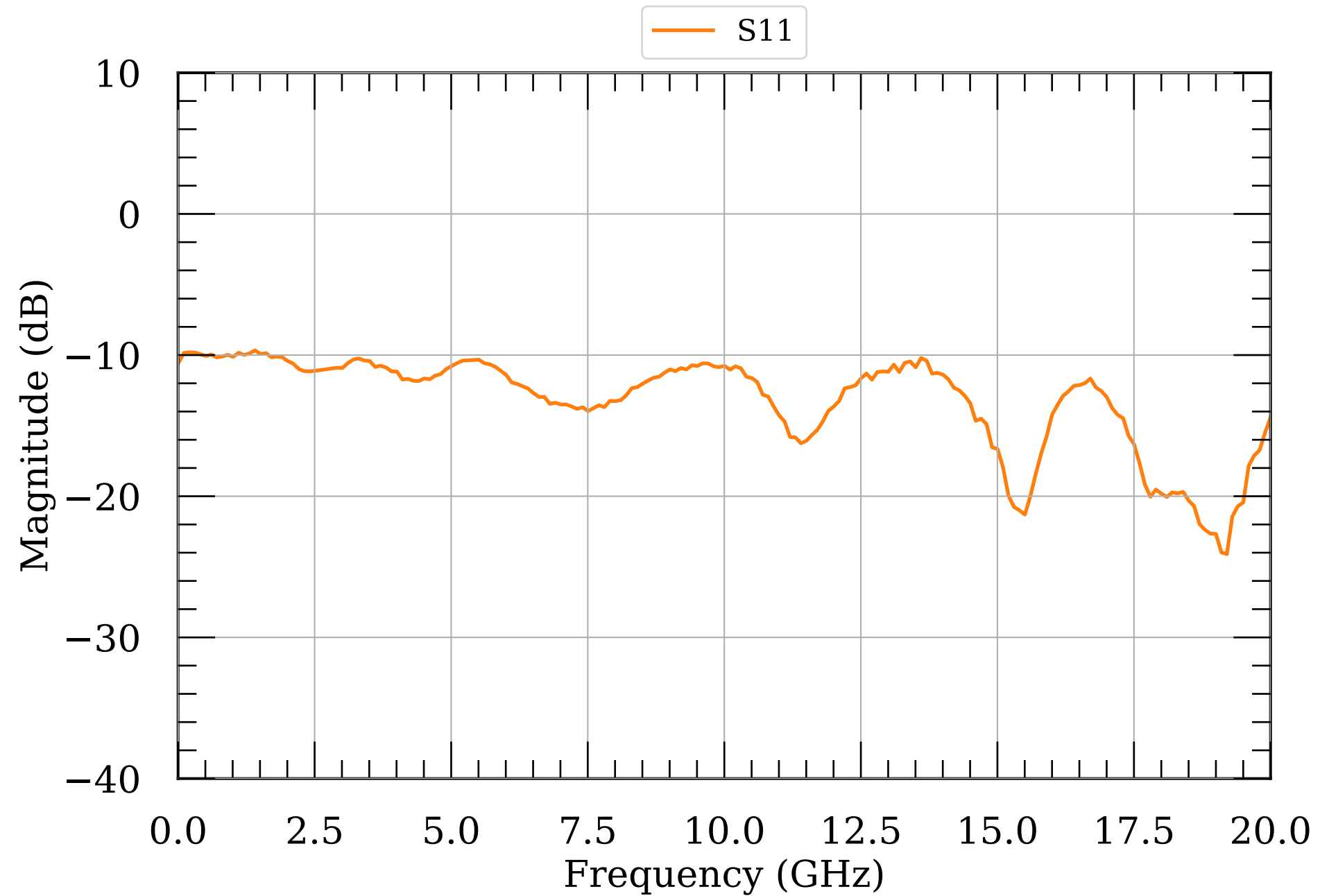
LNA S-params module010v2
